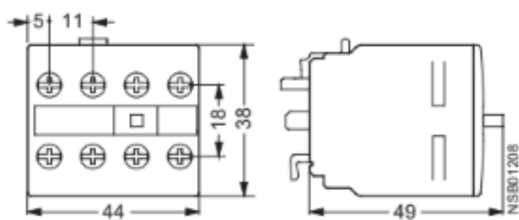
Рис. 2 Габаритные размеры 3RH1921-1FA
