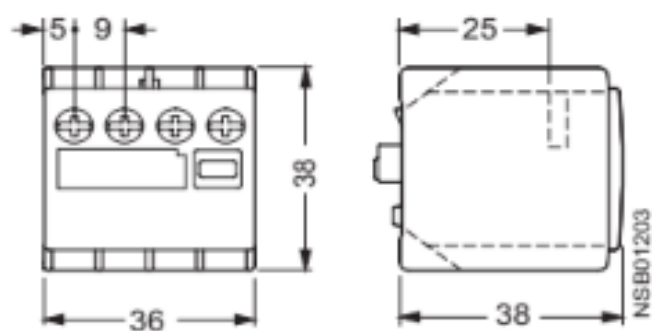
Рис. 1 Габаритные размеры 3RH1911-1FA
